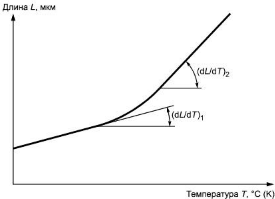
Рисунок 7.1 - Кривая ТМА
