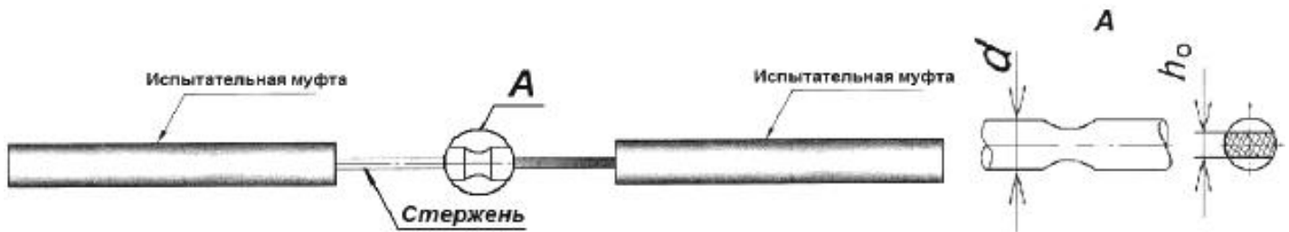
Рисунок Б.1 - Конструкция образца с плоской шейкой
