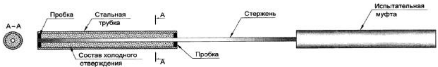
Рисунок 5.1 - Вид типового опытного образца
