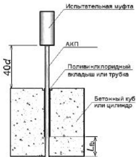
Рисунок 8.1 - Схема образца для испытаний
